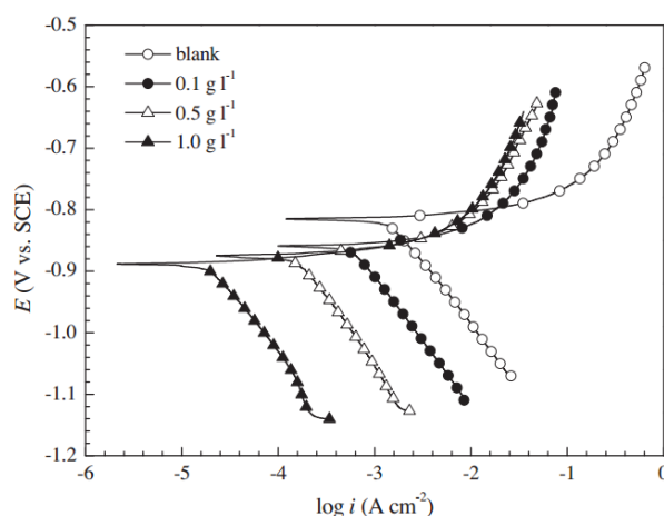
شکل ۳- منحنی تافلای پلاریزاسیون فلز آلومینیم در محیط هیدروکلریک اسید در غیاب و حضور عصاره جیانگ بامبو [۴]
