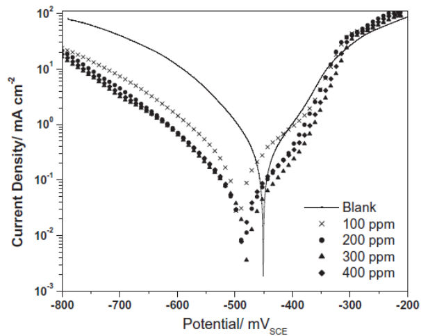
شکل ۸- منحنی پلاریزاسیون فولاد در محیط هیدروکلریک اسید در غیاب و حضور عصاره پوست سیر [۱۵].
