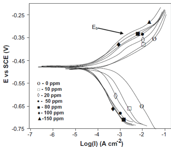
شکل ۴- منحنی تافلای پلاریزاسیون فلز فولاد در محیط هیدروکلریک اسید در غیاب و حضور عصاره گل مشعلی [۵]
