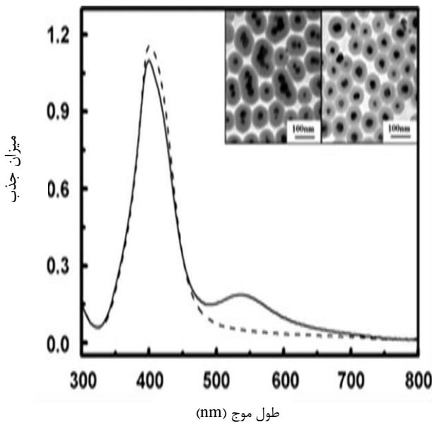
شکل ۲- نتایج طیف سنجی مرئی -فرابنفش نانوذرات نقره قبل (خط تیره) و بعد از استفاده از سیستم استاب (خط چین) [۹].
