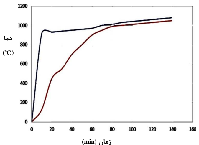
شکل ۳- نمودار دما- زمان برای حریق‌های سلولزی (نمودار قرمز) و حریق‌های هیدروکربنی (نمودار سیاه) [۲۵].
