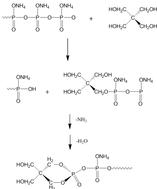
شکل ۲- واکنش بین پلی فسفات آمونیم، به عنوان تولیدکننده اسید، و پنتاریتریتول، به عنوان تولیدکننده کربن [۲۳].
