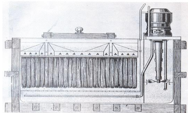
شکل ۶- دستگاه رنگری کلاف [۳۰].
