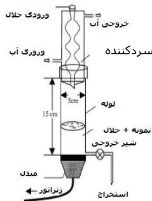
شکل ۳- دستگاه استخراج با کمک امواج فراصوت [۱۲].
