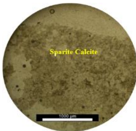
شکل ۸: تصویر میکروسکوپی نمونه C-1، نور PPL، بزرگنمایی 4X، تصویر شماره ۷ در نور پلاریزه. در این نور کلسیت اسپارایتی به رنگ روشن و شفاف دیده می‌شود. Figure 8: Microscopic image of sample C-1, PPL light, 4X magnification, image 7 in polarized light. In this light, sparite calcite can be seen in a bright and transparent color.
