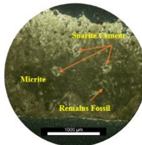
شکل ۵: تصویر میکروسکوپی نمونه B-4، نور XPL، بزرگنمایی 4X، نمونه متشکل از کلسیت میکرایتی است. بقایای از قطعات فسیل و کلسیت ثانویه (سیمان اسپرایتی) در تصویر دیده می‌شود.
