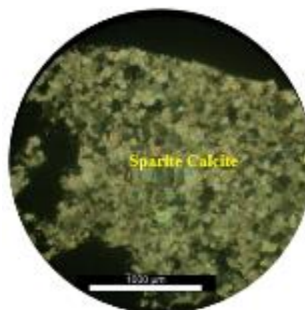
شکل ۷: تصویر میکروسکوپی نمونه C-1، نور XPL، بزرگنمایی 4X، نمونه تماماً از کلسیت درشت بلور یا اسپارایت تشکیل شده است. Figure 7: Microscopic image of sample C-1, XPL light, 4X magnification, the sample is entirely composed of coarse calcite or sparite.
