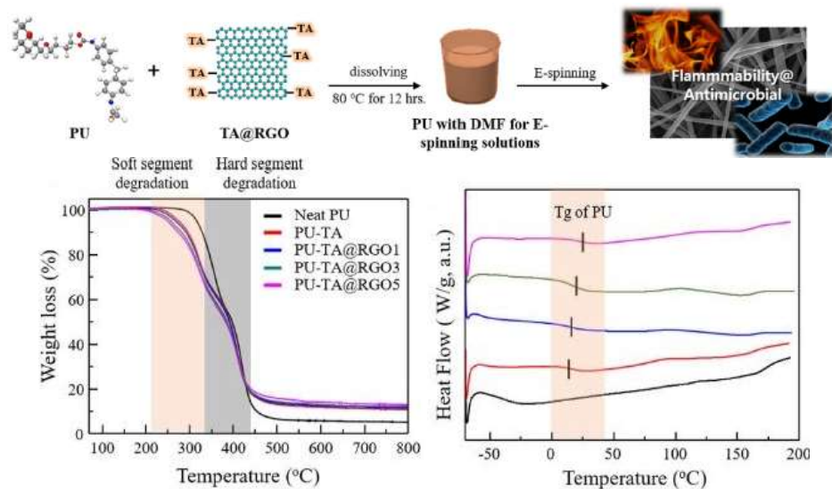
شکل ۳: شیمیایی از سنتز و نمودار TGA و DSC نمونه‌های آماده شده از TA@RGO (۱۸).
