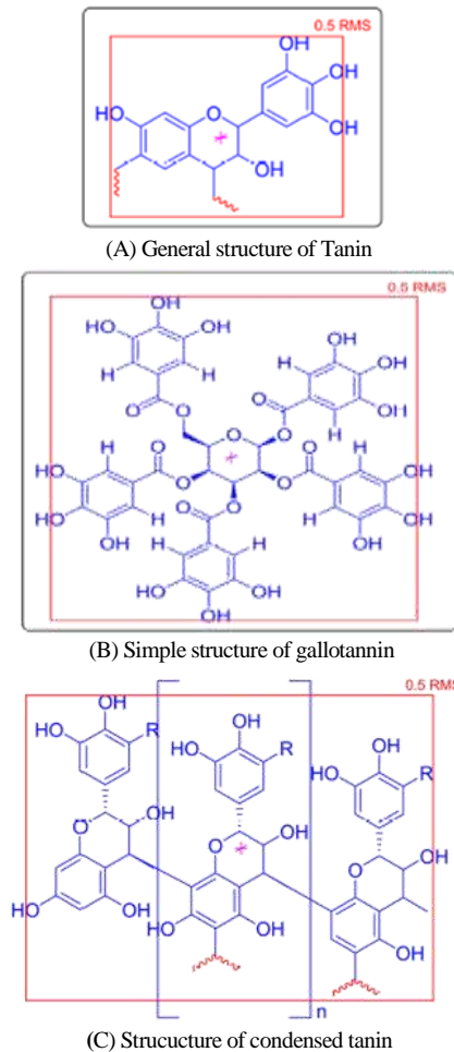
شکل ۲: ساختار شیمیایی تانن‌ها و اسید تانیک (۱۵).
