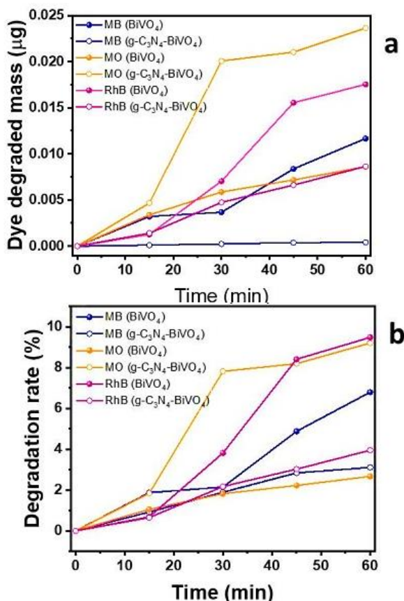
شکل ۲: (a) جرم رنگ‌زای تخریب شده به عنوان تابع از زمان، و (b) میزان تخریب به عنوان تابع از زمان، با استفاده از BiVO_4 و g-C_3N_4/BiVO_4 به عنوان جاذب و رنگ‌ها: متیلن بلو (MB)، متیل اورانژ (MO) و رودامین بی (RhB) با مقدار ۳۰ mg/L قبل از جذب (۳۲).
