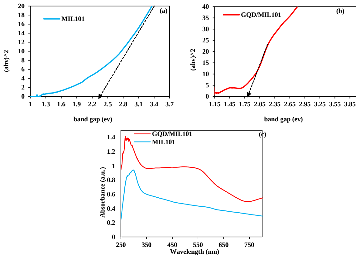
شکل ۴: محاسبه گاف نوار از طریق روش نمودار Tauc برای (a) MIL-101 (Fe)، (b) MIL-101/GQD، و (c) تجزیه و تحلیل UV-vis/DRS برای MIL-101 (Fe) و MIL-101/GQD.
