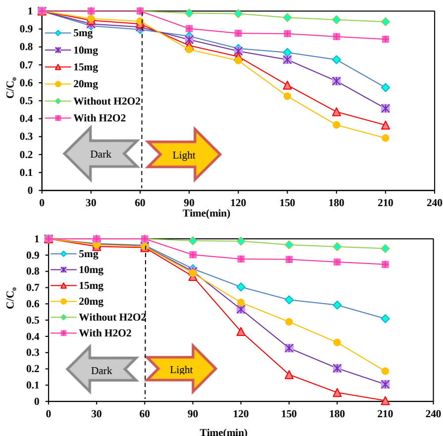
شکل ۱۰: مقایسه عملکرد مقادیر مختلف کامپوزیت GQD/MIL101، در ۱۰۰ میلی لیتر محلول ۲۰ میلی گرم بر لیتر مالاکیت سبز، تحت تابش نور مرئی ۳ pH و ۲ \mu\text{L} \text{H}_2\text{O}_2 .
